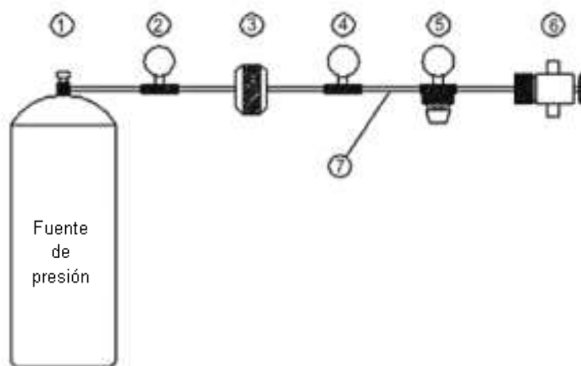
Figura 1 - Dispositivo de ensayo de medición entre caudal máximo y caudal residual
